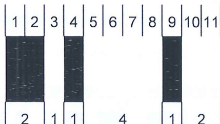
Hình 11 – Ký tự xác định bắt đầu A của mã vạch 128
